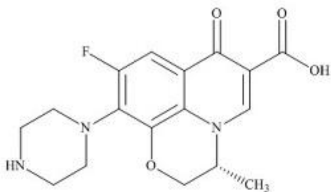
左氧氟沙星杂质 29
