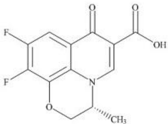
左氧氟沙星杂质 8
