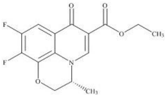
左氧氟沙星杂质 9
