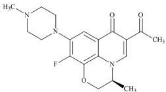
左氧氟沙星杂质 20
